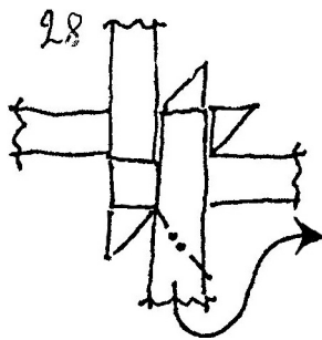
Согнуть «горой».
